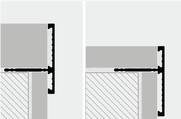
ESEMPI DI POSA - INSTALLATION EXAMPLES EXEMPLES DE POSE - VERLEGEBEISPIELE
