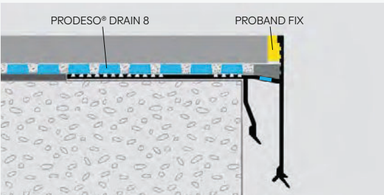
ESEMPI DI POSA - INSTALLATION EXAMPLES EXEMPLES DE POSE - VERLEGEBEISPIELE
