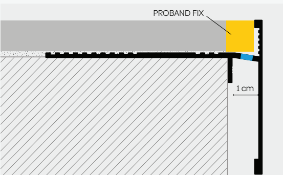
ESEMPI DI POSA - INSTALLATION EXAMPLES EXEMPLES DE POSE - VERLEGEBEISPIELE
